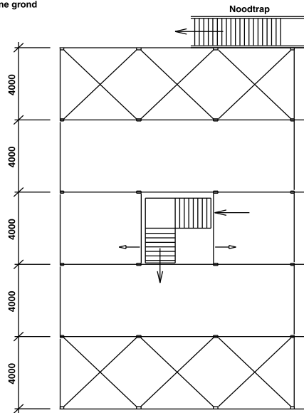
Begane grond
